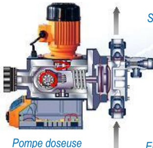
Pompe doseuse
